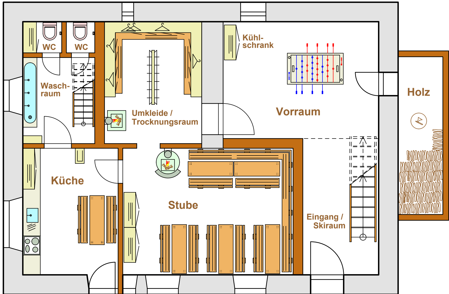
Erdgeschoss 1:50
